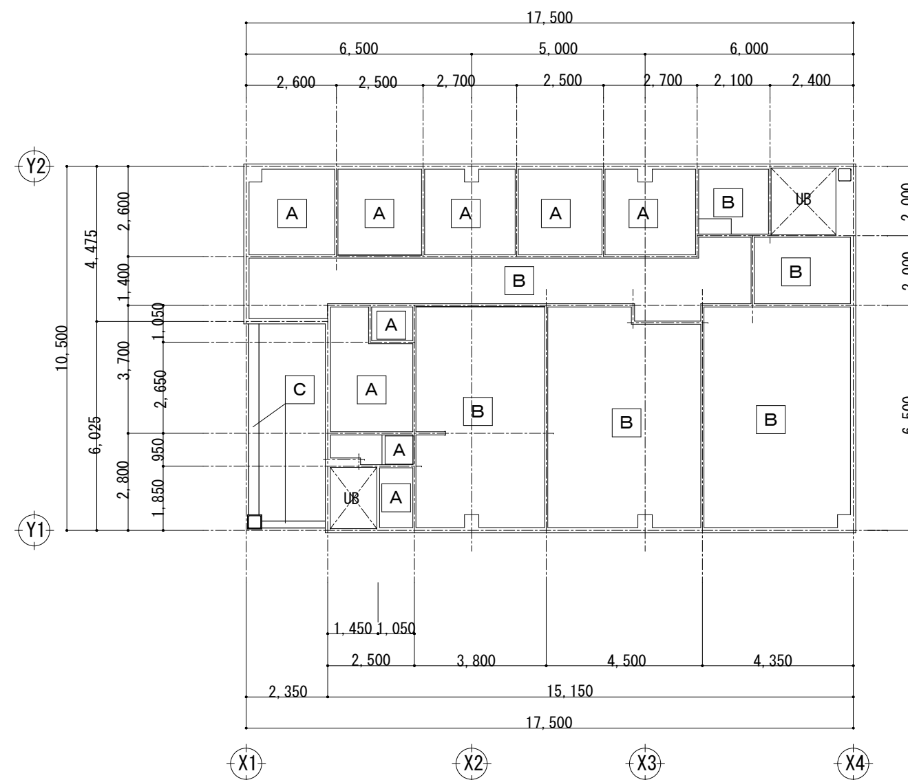
2階天井伏図 S=1/150
