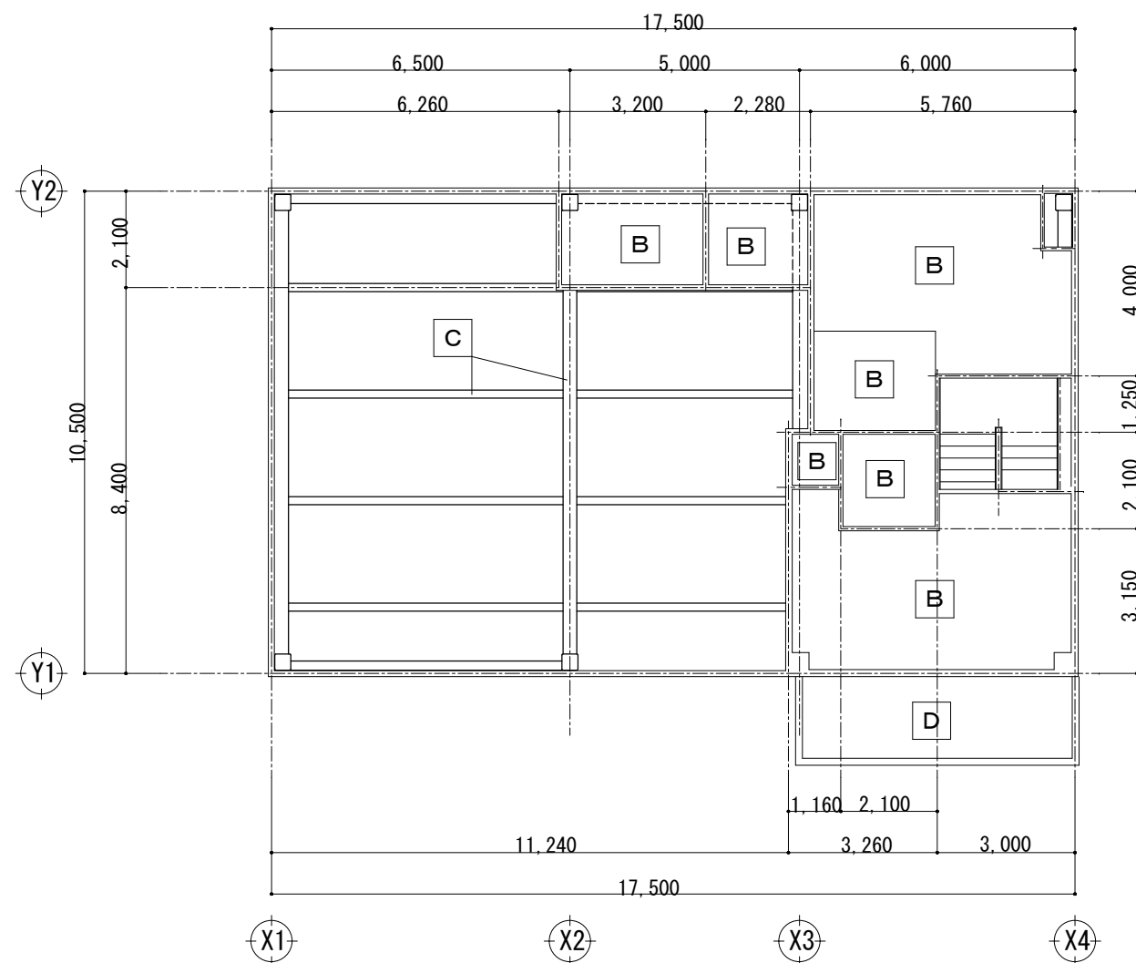
1階天井伏図 S=1/150
